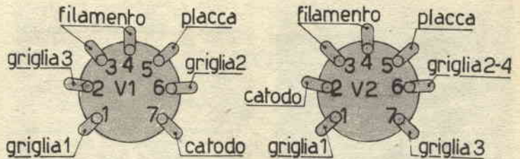
Fig.1 - CONNESSIONI ALLO ZOCCOLO
