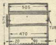
DETTAGLIO DEL CILINDRO ESTERNO E DEL VASSOIO
