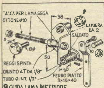
9 GUIDA LAMA INFERIORE
