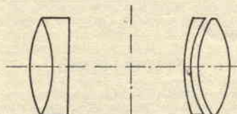
SCHEMA OBIETTIVO PETZVAL
